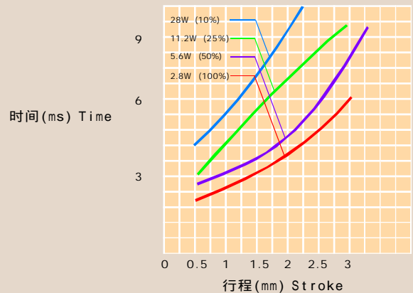
行程/应答时间 Stroke and Time
